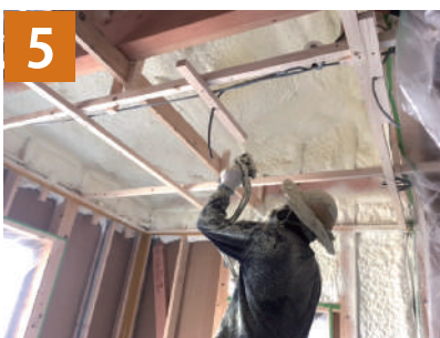
母屋の上にサーモバリアエアーを敷き、タルキを取付け通気層を確保し、 発泡ウレタンをサーモバリアエアーに吹付けます。
